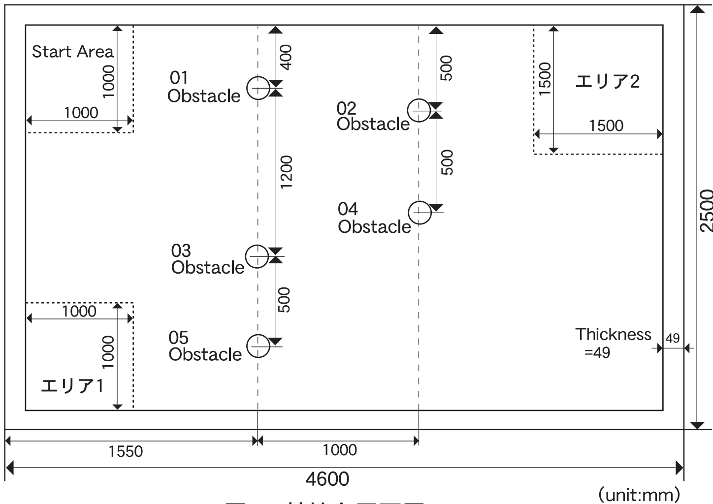
図1：競技台平面図
